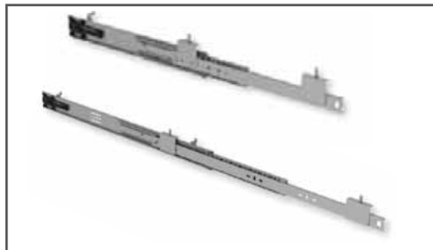
Telescopic slides - 40cm or 60cm deep BBG-RK-E/U
